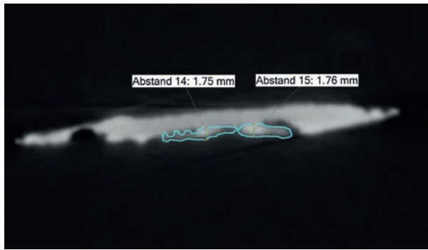
Abb. 9 Querschnitt der Inschrift im Bereich des ersten Kreuzes mit Begrenzungsmarkierung und Vermessung.
