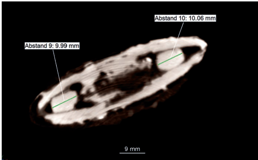
Abb. 14 Querschnitt und Durchmesser des Bügels.
